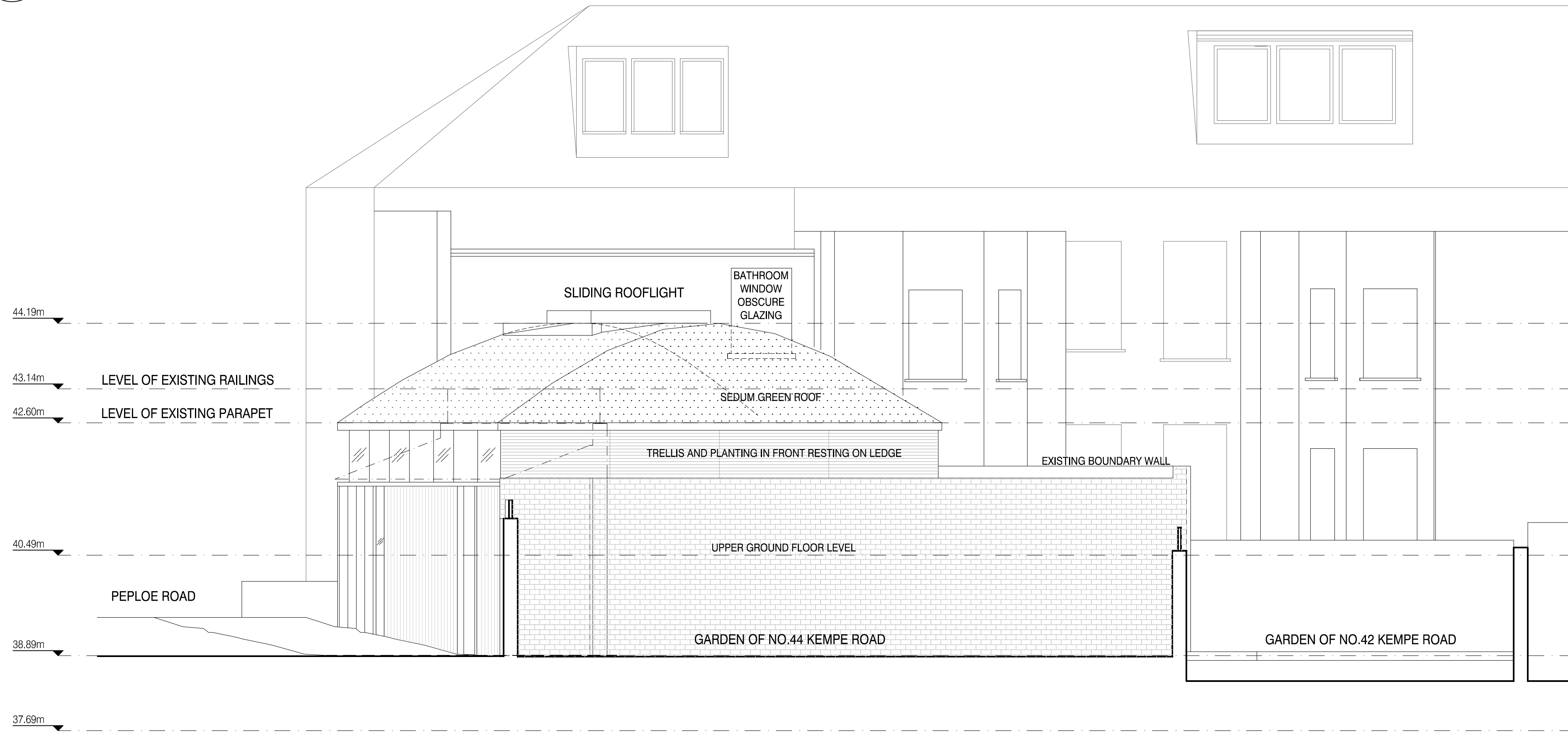
01 ELEVATION A SCALE: 1:100@A3
