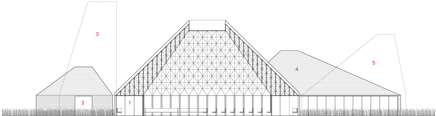
Section A-A
